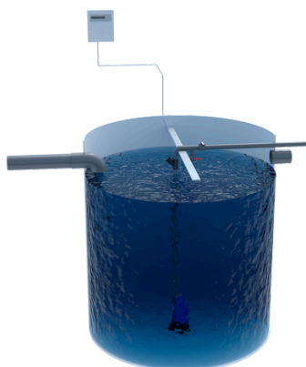
POZO DE BOMBEO
